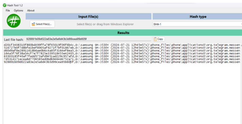
Gambar 10. Proses Validasi Barang Bukti
